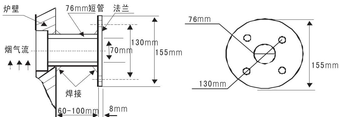
接管法兰与炉体的连接示意图
